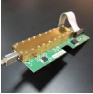
250MHz-20GHz RF Module (U6200-opt02).
